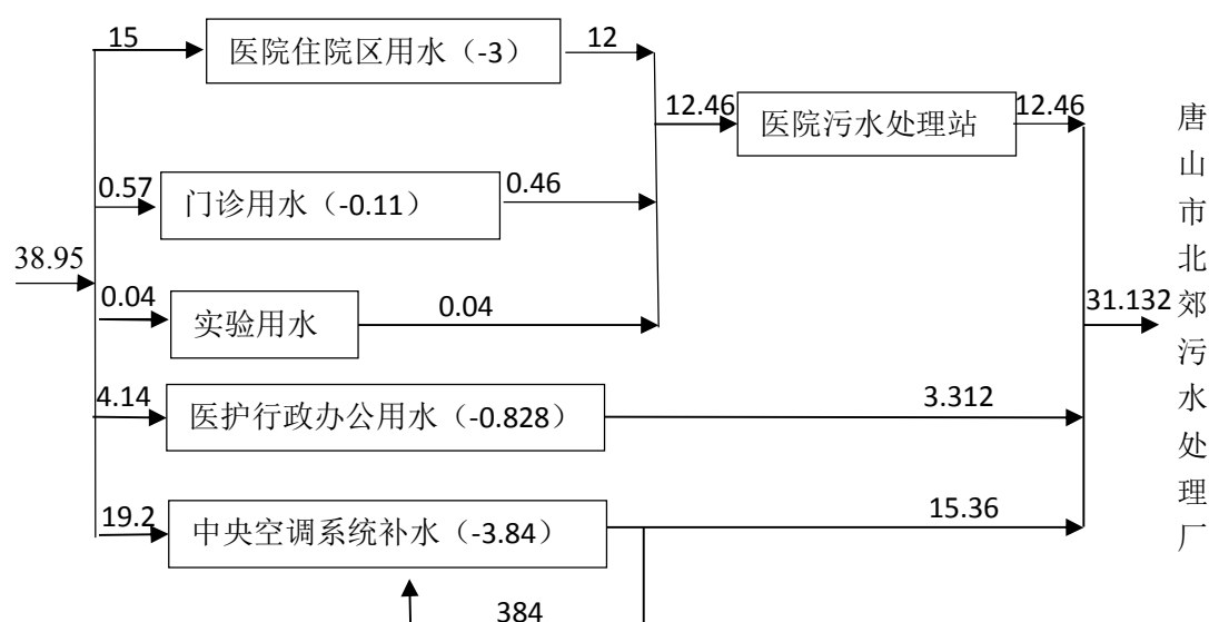
图 2 项目扩建后全院水平衡图 \text{m}^3/\text{d}
